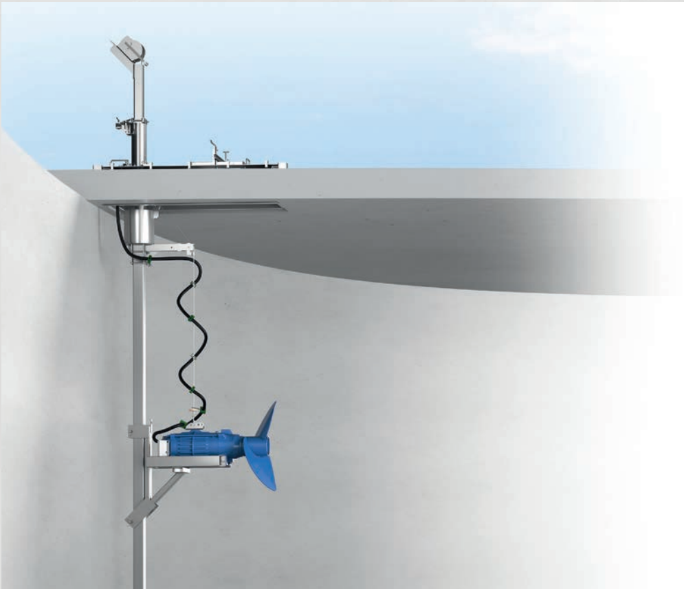
Abbildung EGR 4 (Service-Deckel) mit GTWSB 204
