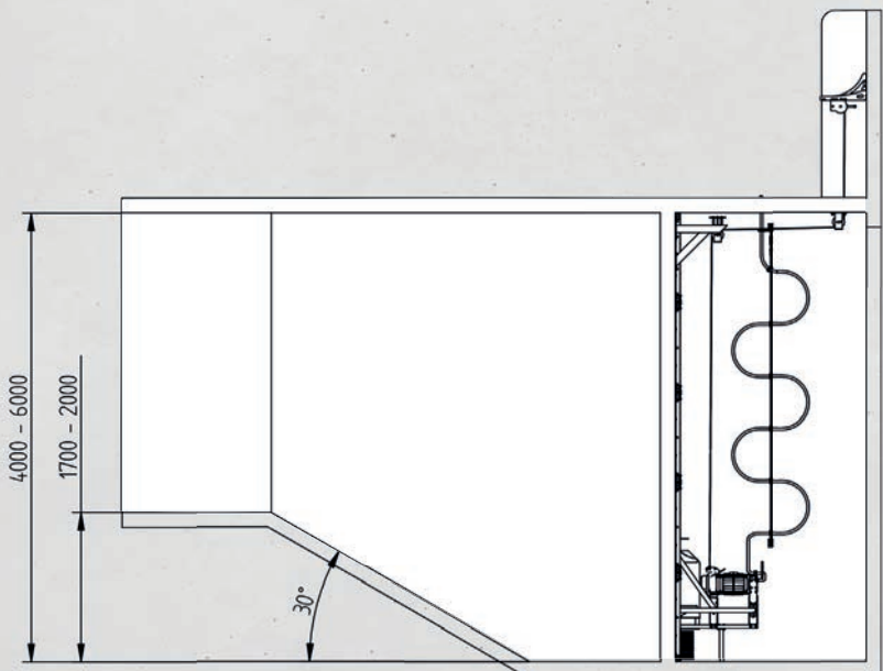
Abbildung: Einbaumaße
